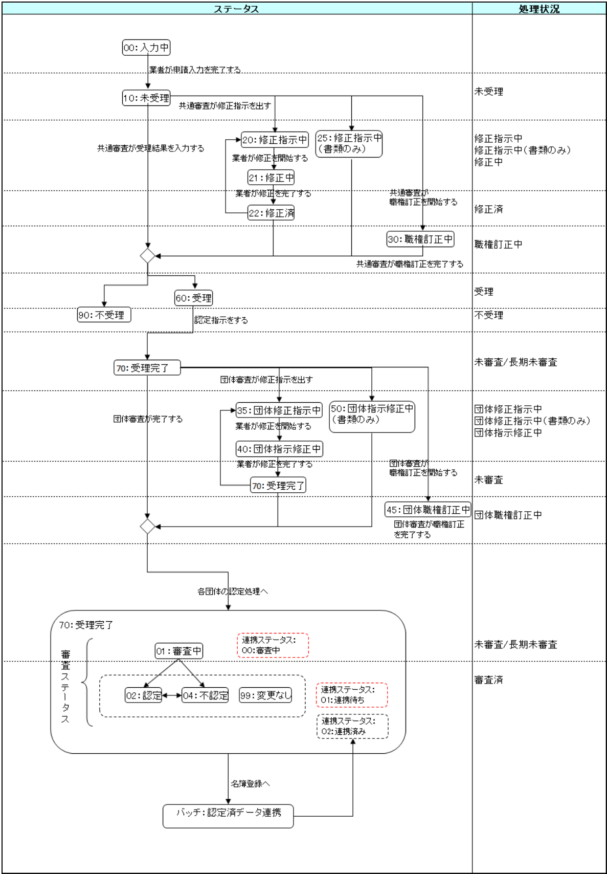
検索条件「処理状況」と申請に対する各アクションの関係図
